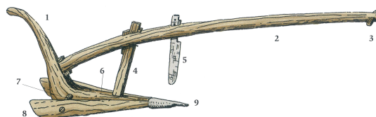
Partes del arado. 1. Mancera; 2. Timón; 3. Clavija; 4. Teiruga; 5. Seita; 6. Rostro; 7. Amexelo; 8. Abeacas; 9. Rella
